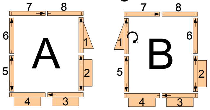
Plan de montage des chalets
